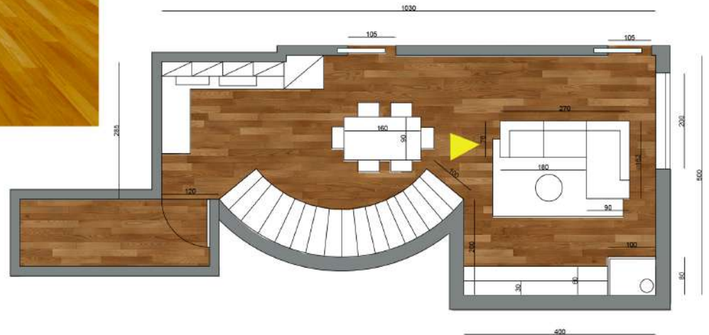
PLANIMETRIA PROGETTO
