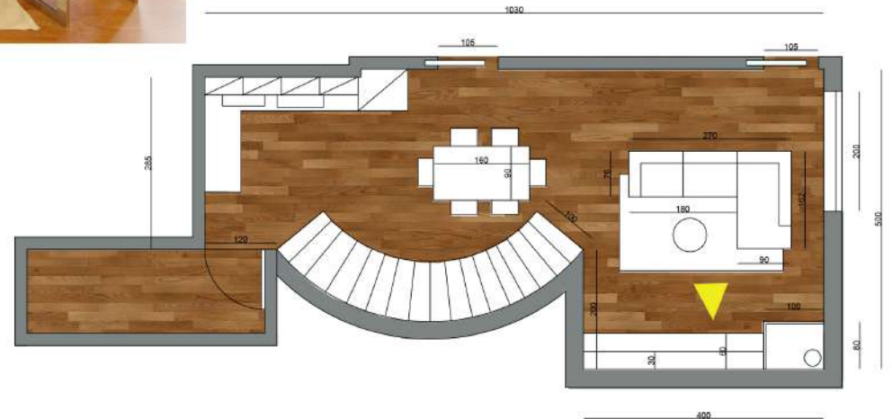
PLANIMETRIA PROGETTO
