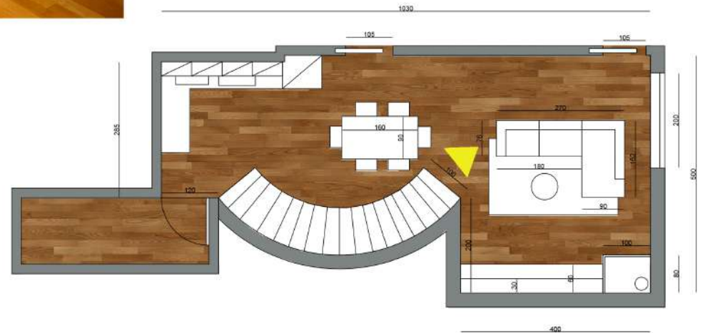
PLANIMETRIA PROGETTO
